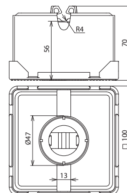
Beépítési méretek
