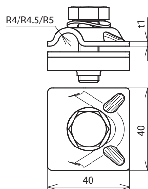
Beépítési méretek
