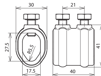
Beépítési méretek
