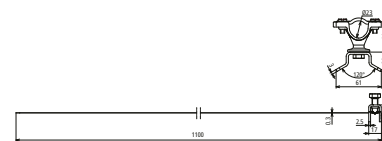
Beépítési méretek
