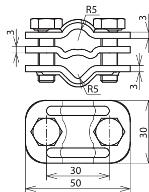
Beépítési méretek
