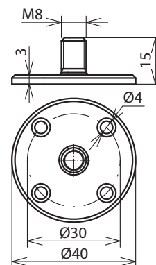
Beépítési méretek
