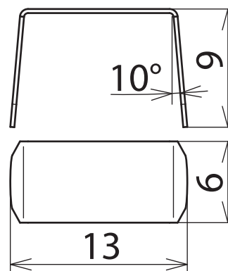
Beépítési méretek
