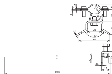
Beépítési méretek
