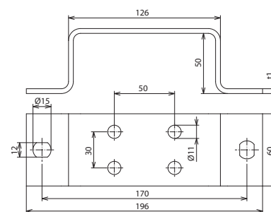
Beépítési méretek
