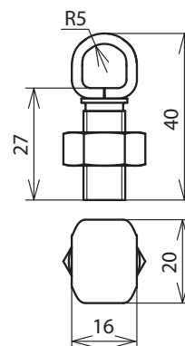
Beépítési méretek
