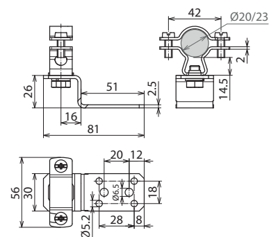
Beépítési méretek
