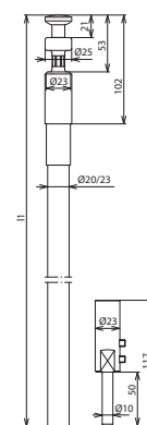
Beépítési méretek
