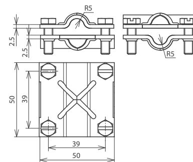
Beépítési méretek
