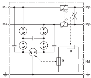
Kapcsolási rajz
