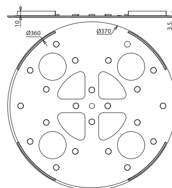
Beépítési méretek
