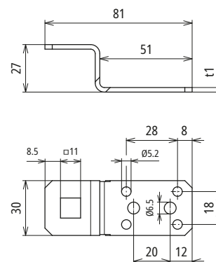
Beépítési méretek
