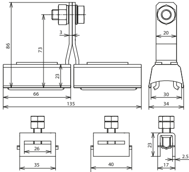
Beépítési méretek
