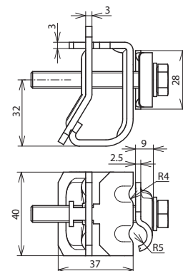
Beépítési méretek
