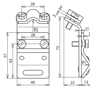
Beépítési méretek
