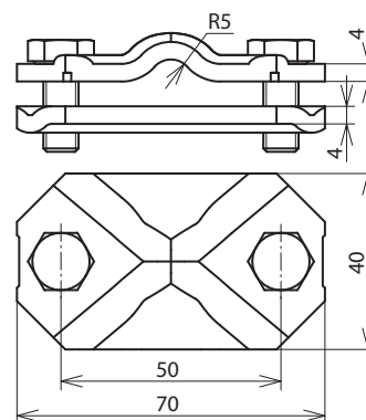
Beépítési méretek
