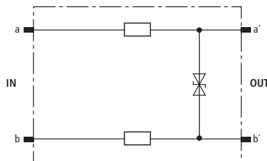
Kapcsolási rajz
