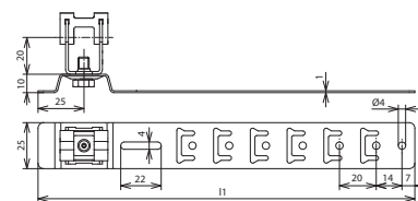
Beépítési méretek
