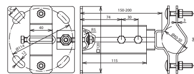
Beépítési méretek
