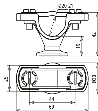
Beépítési méretek
