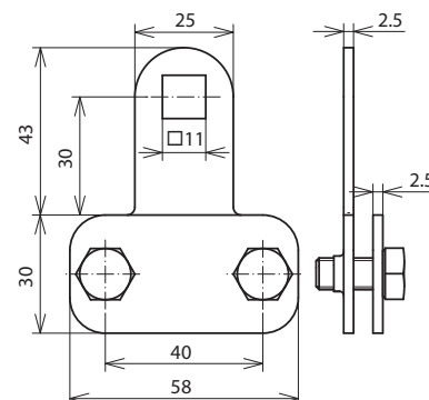
Beépítési méretek
