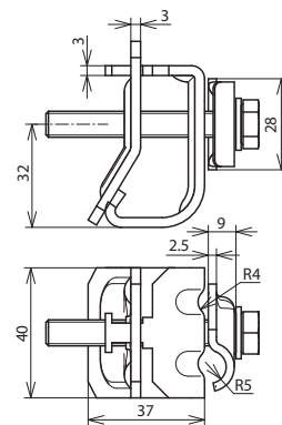
Beépítési méretek
