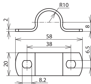
Beépítési méretek
