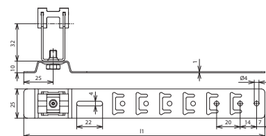
Beépítési méretek
