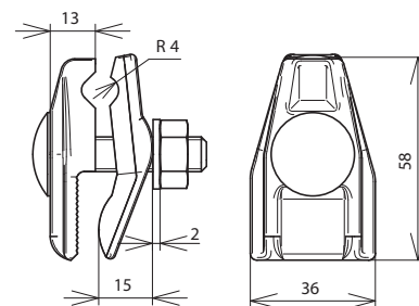
Beépítési méretek
