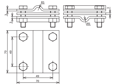
Beépítési méretek
