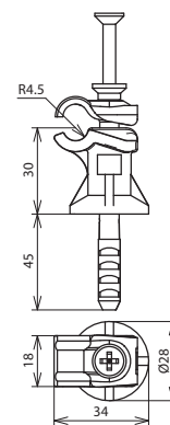
Beépítési méretek
