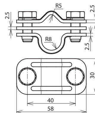
Beépítési méretek
