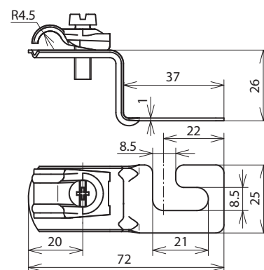
Beépítési méretek
