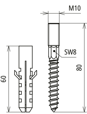
Beépítési méretek
