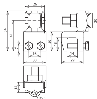
Beépítési méretek
