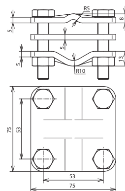
Beépítési méretek
