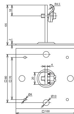
Beépítési méretek
