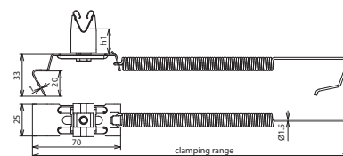
Beépítési méretek
