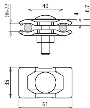
Beépítési méretek
