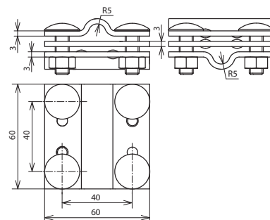
Beépítési méretek
