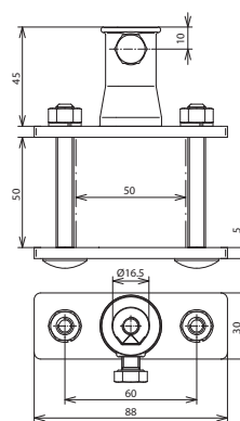
Beépítési méretek
