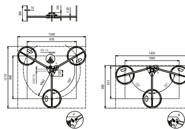
Beépítési méretek
