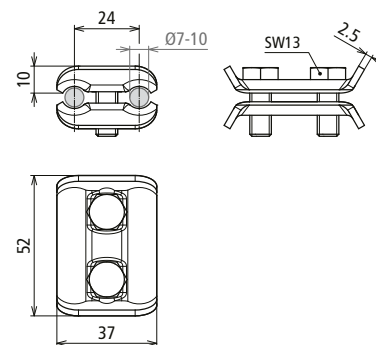
Beépítési méretek
