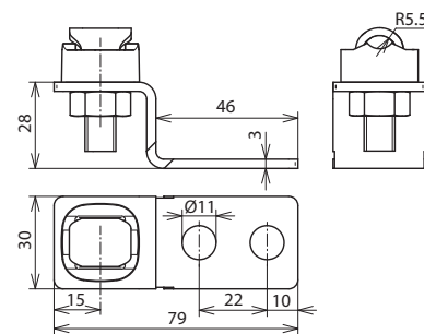
Beépítési méretek
