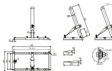
Beépítési méretek
