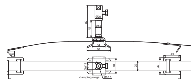
Beépítési méretek
