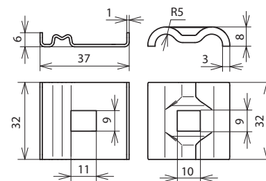
Beépítési méretek
