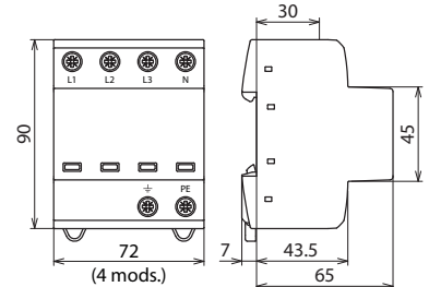
Beépítési méretek
