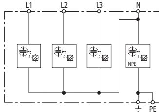
Kapcsolási rajz
