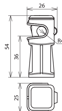
Beépítési méretek
