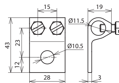
Beépítési méretek
